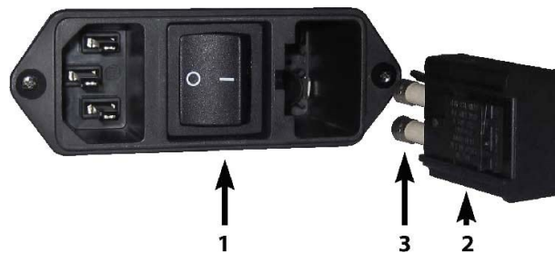
ABB 5-4 STROMEINGANGSBAUTEIL
