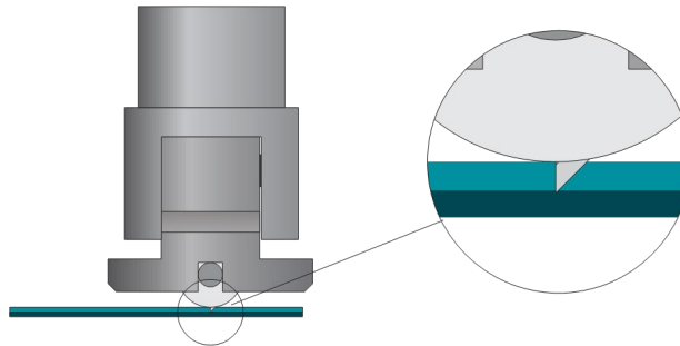
FIG 2-10 EINSTELLUNG MESSERTIEFE NORMALES SCHNEIDEN
