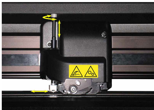
ABB 1-28 ENTFERNEN DES TANGENTIALEN MESSERHALTERS
