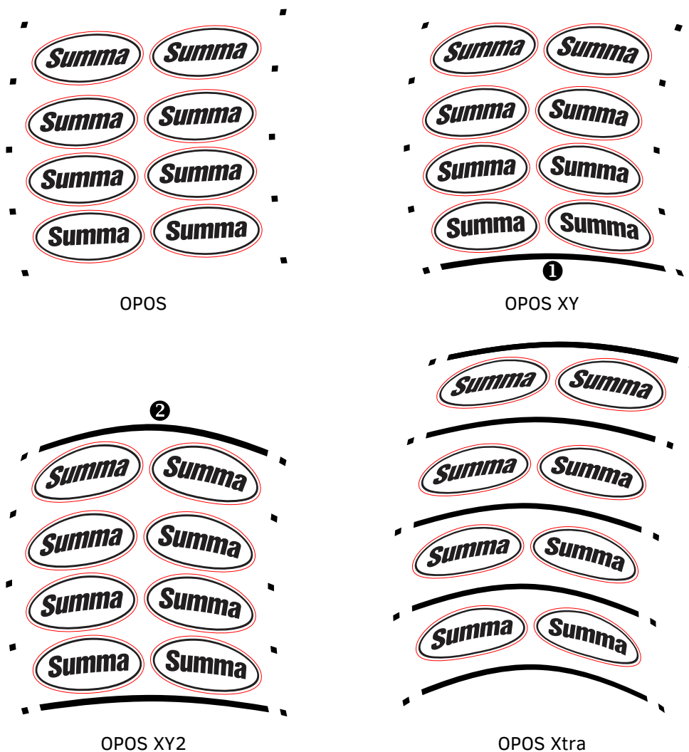
FIG 3-3 OPOS-AUSRICHTUNGSMETHODEN
