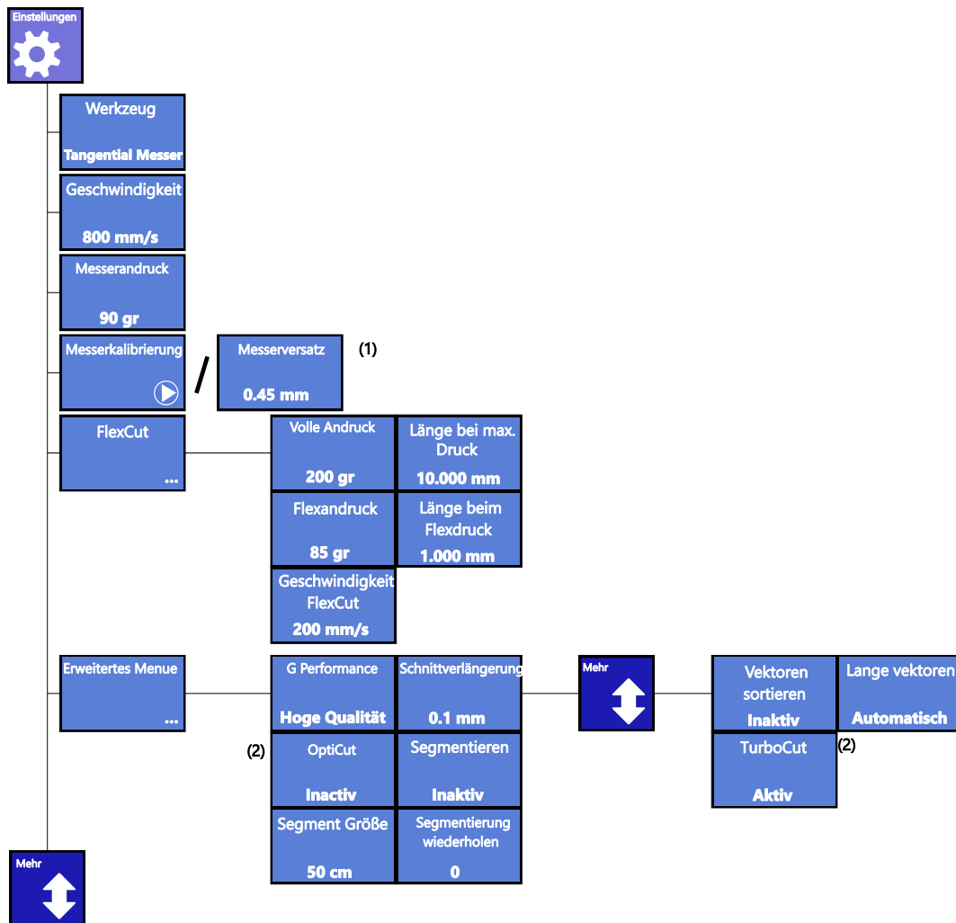
ABB 4-2 EINSTELLUNGEN MENÜ
