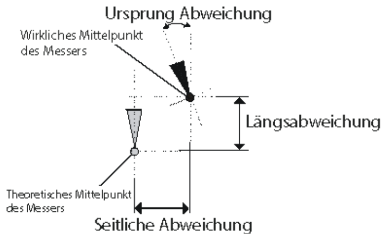
ABB 2-5 MÖGLICHE MESSERKALIBRIERUNG
