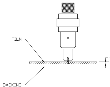
ABB 1-25 ANPASSUNG MESSERLÄNGE
