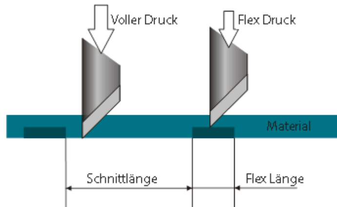
ABB 2-8 FLEXCUT PRINZIP
