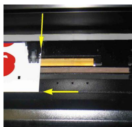
ABB 3-4 POSITION DES MATERIALS FÜR MEHRERE BLÄTTER
