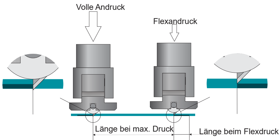
FIG 2-11 EINSTELLUNG MESSERTIEFE DURCHSCHNEIDEN
