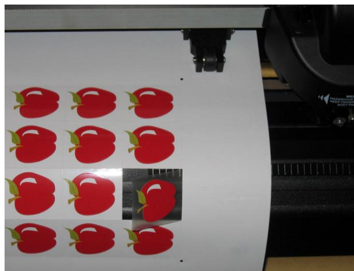
ABB 2-9 KOMBINIERTES KONTURSCHNEIDEN UND DURCHSCHNEIDEN
