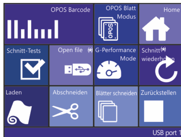
ABB 4-1 AKTIONEN-MENÜ
