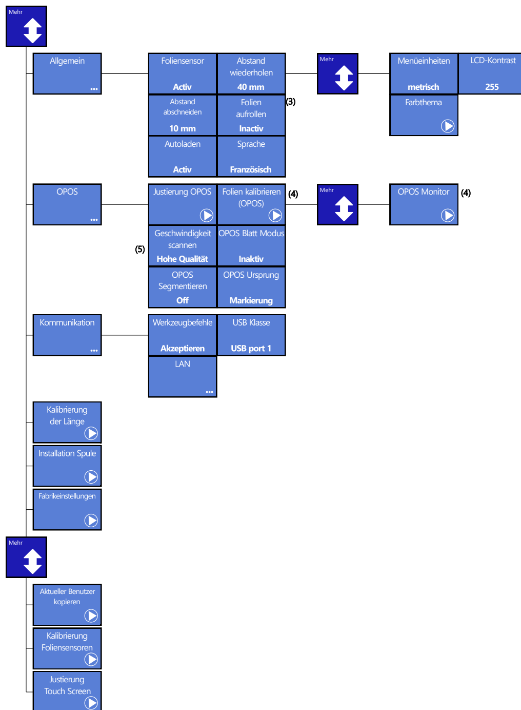
ABB 4-3 EINSTELLUNGEN MENÜ
