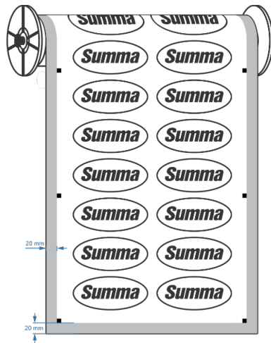
FIG 3-1 RÄNDER FÜR DEN DRUCK AUF ROLLE
