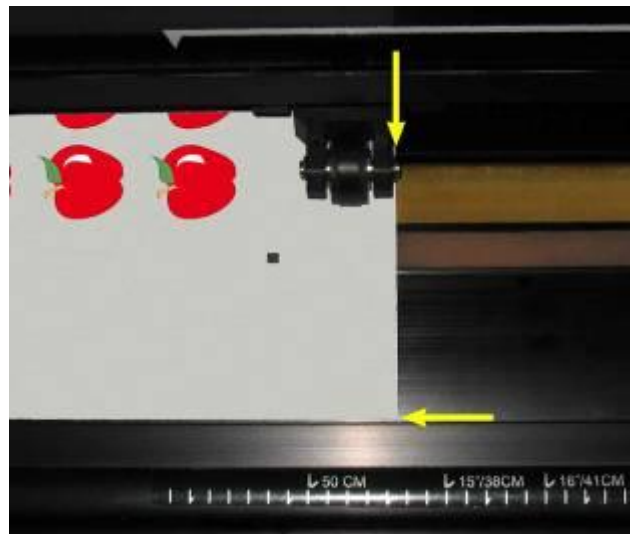
FIGURA 3-1 POSIÇÃO DO MATERIAL PARA MÚLTIPLAS FOLHAS
