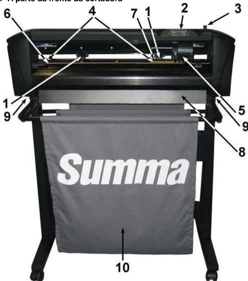
FIGURA 1-10 A PARTE DA FRENTE DA CORTADORA SUMMACUT
