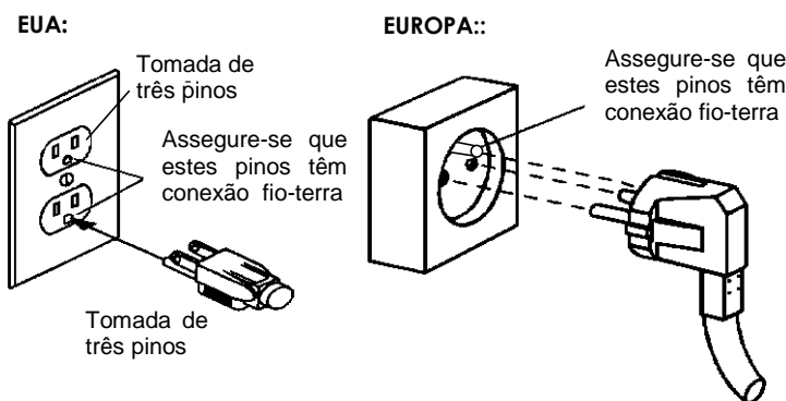
FIGURA 1-12 CONEXÃO ADEQUADA DO FIO-TERRA
