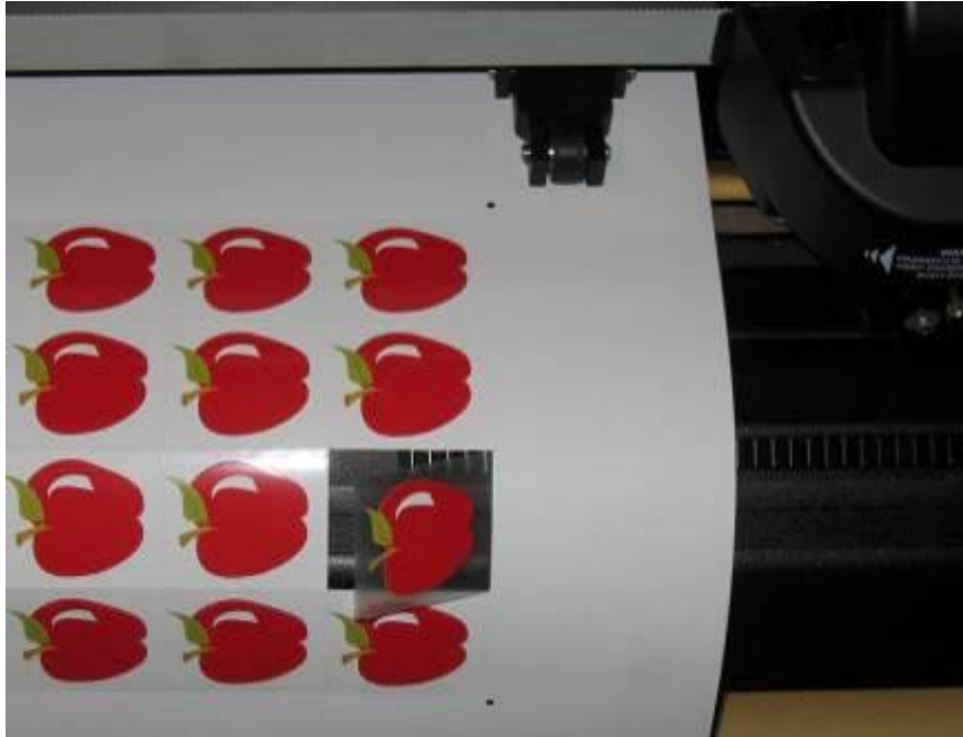
FIGURA 3-4 CORTE SIMULTÂNEO DE CONTOURO E PERFURAÇÃO
